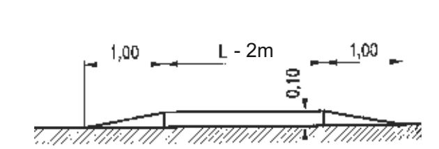
Przekrój progu U-16c
