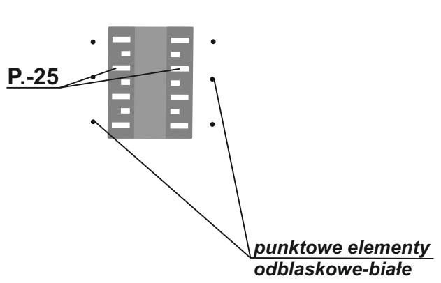
Wzór oznakowania progu
